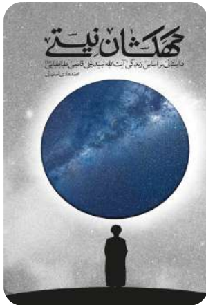
کَهکشان نیستی
